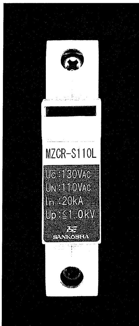
图 1 样品照片
